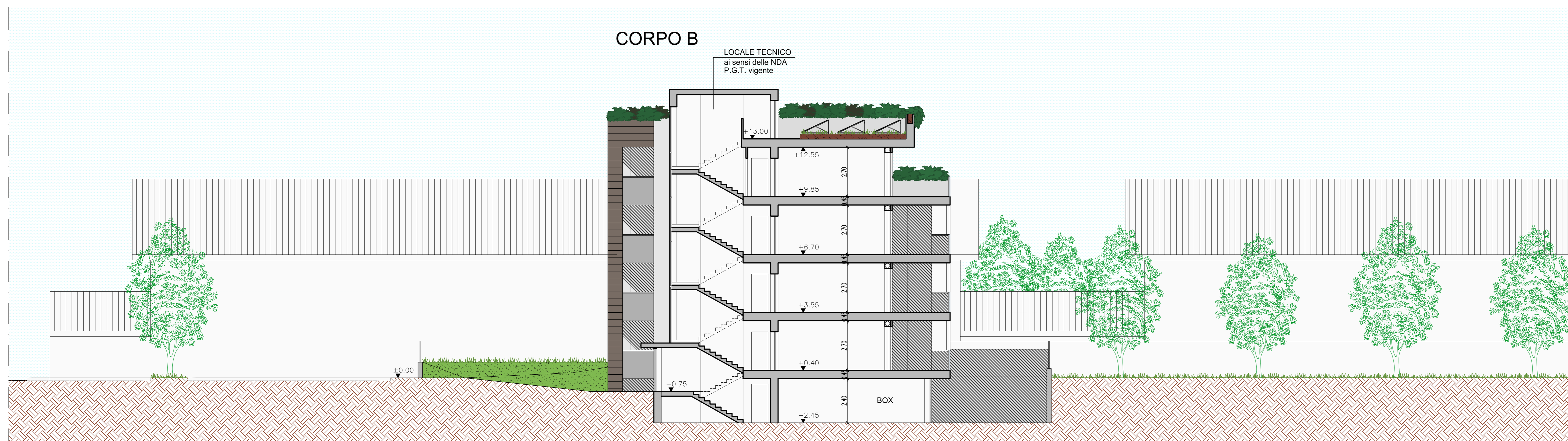
SEZIONE TIPO - CORPO B
