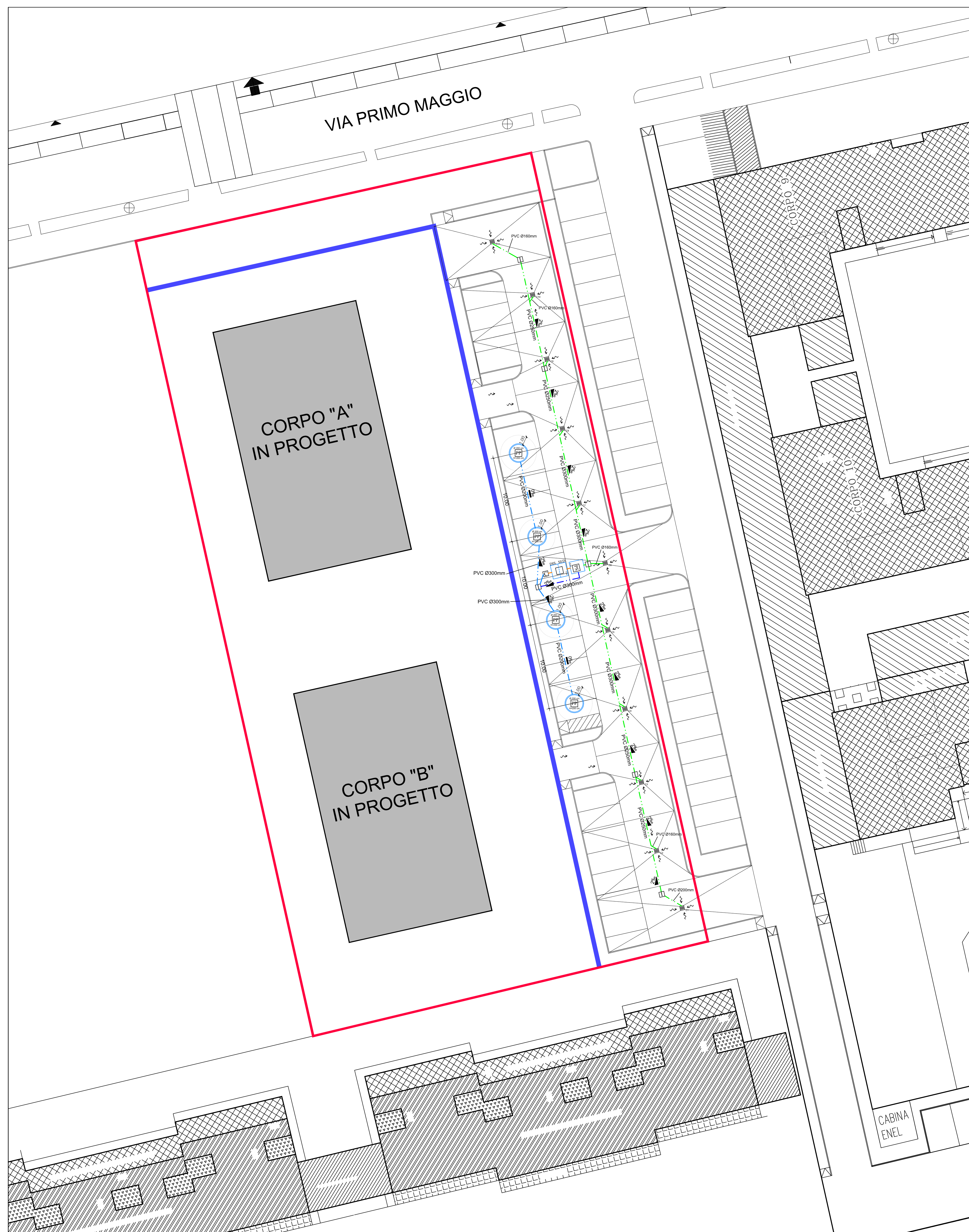
NORD PLANIMETRIA GENERALE URBANIZZAZIONI - SMALTIMENTO ACQUE METEORICHE Scala 1:200
