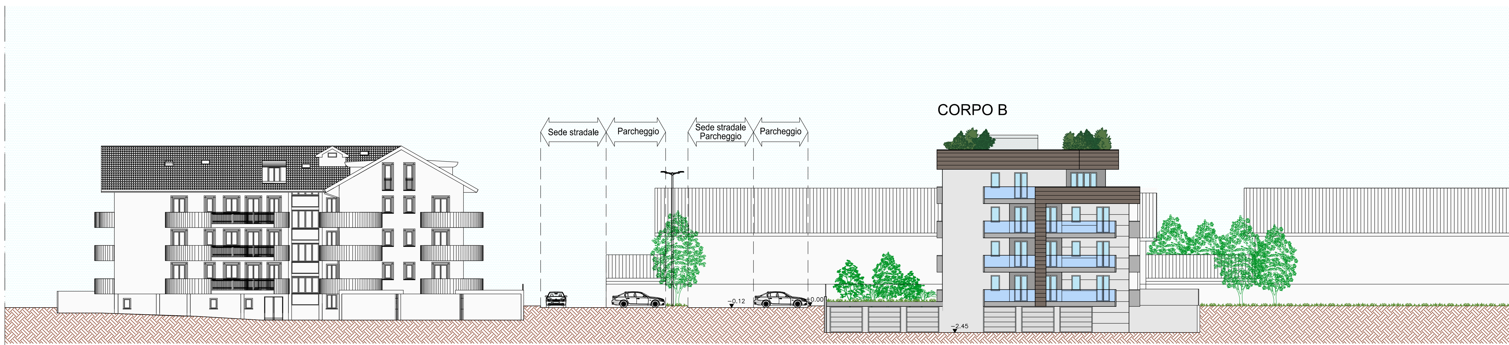
STATO DI PROGETTO - SEZIONE A-A Scala 1:200
