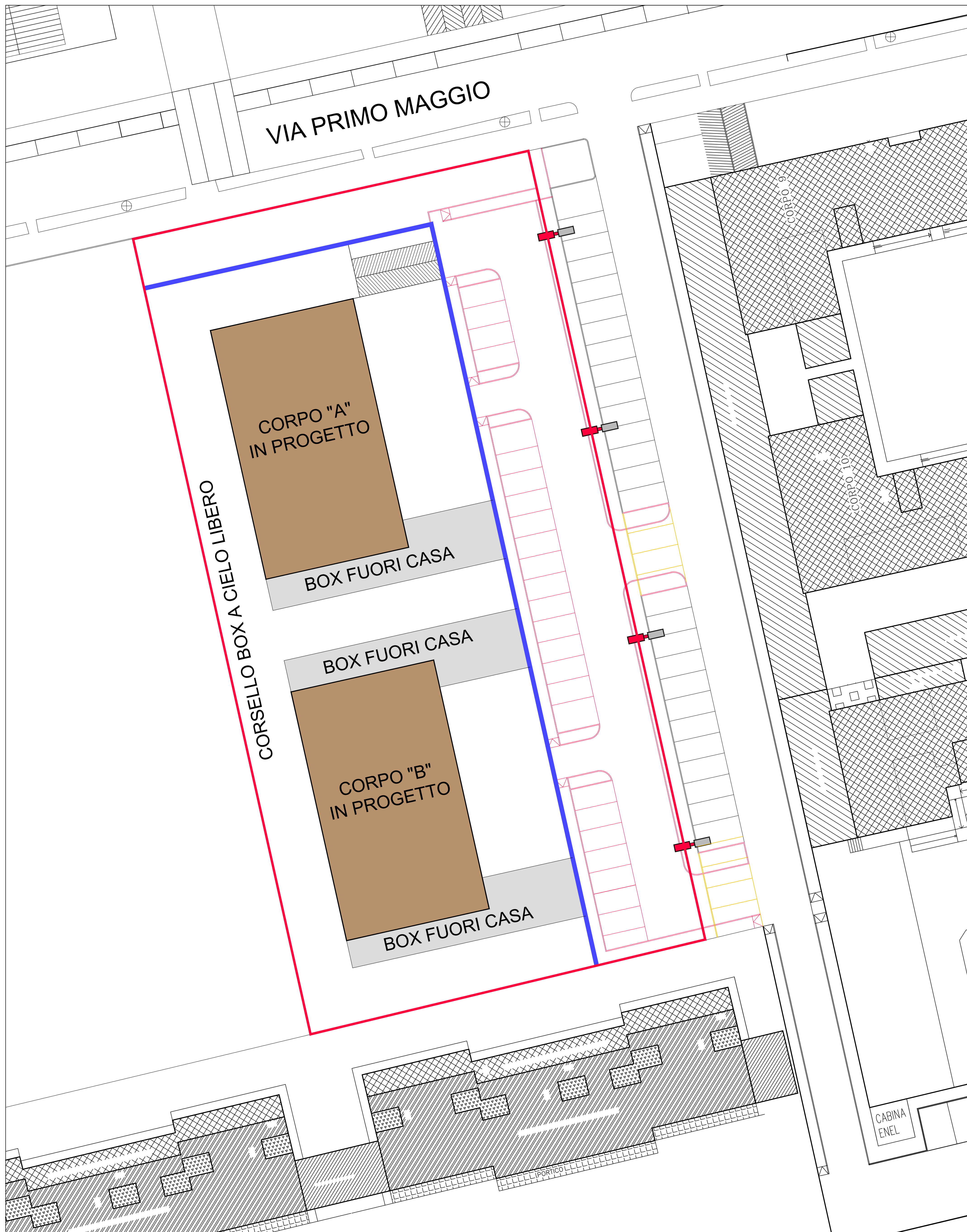
PLANIMETRIA GENERALE URBANIZZAZIONI - STATO DI CONFRONTO Scala 1:500
