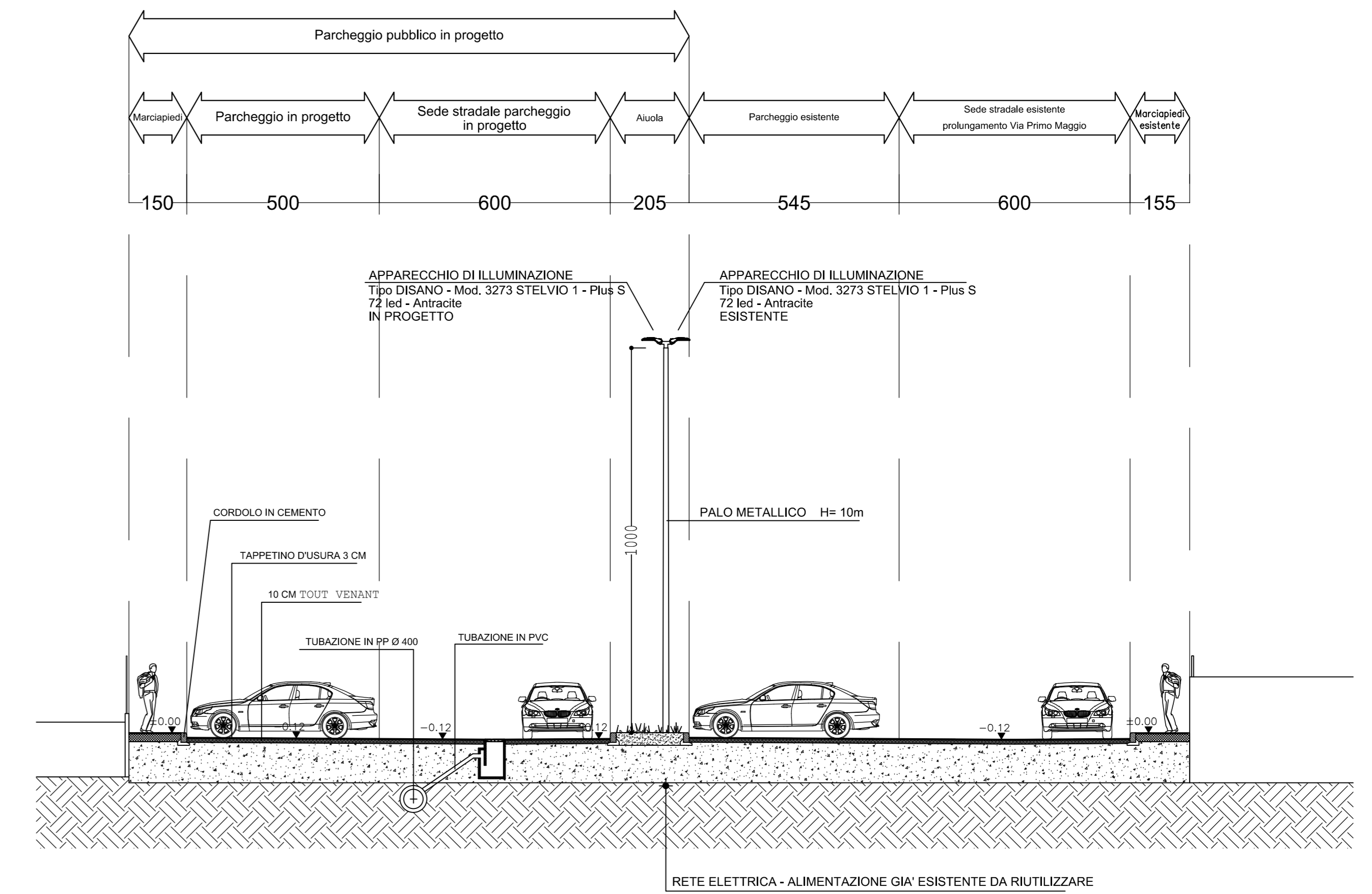
STATO DI PROGETTO - SEZIONE A-A Scala 1:100
