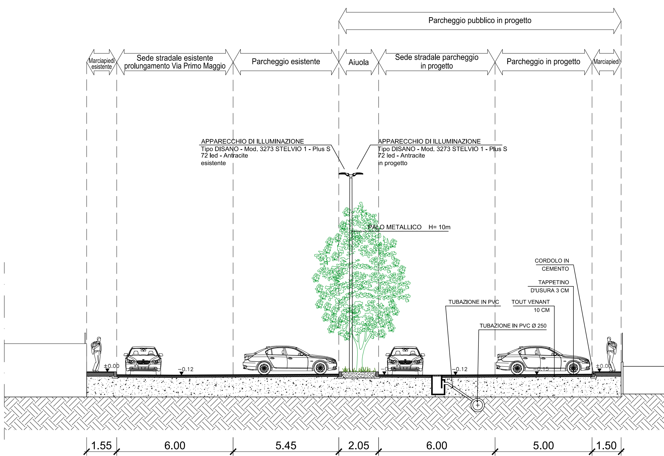
STATO DI PROGETTO - SEZIONE A-A Scala 1:100
