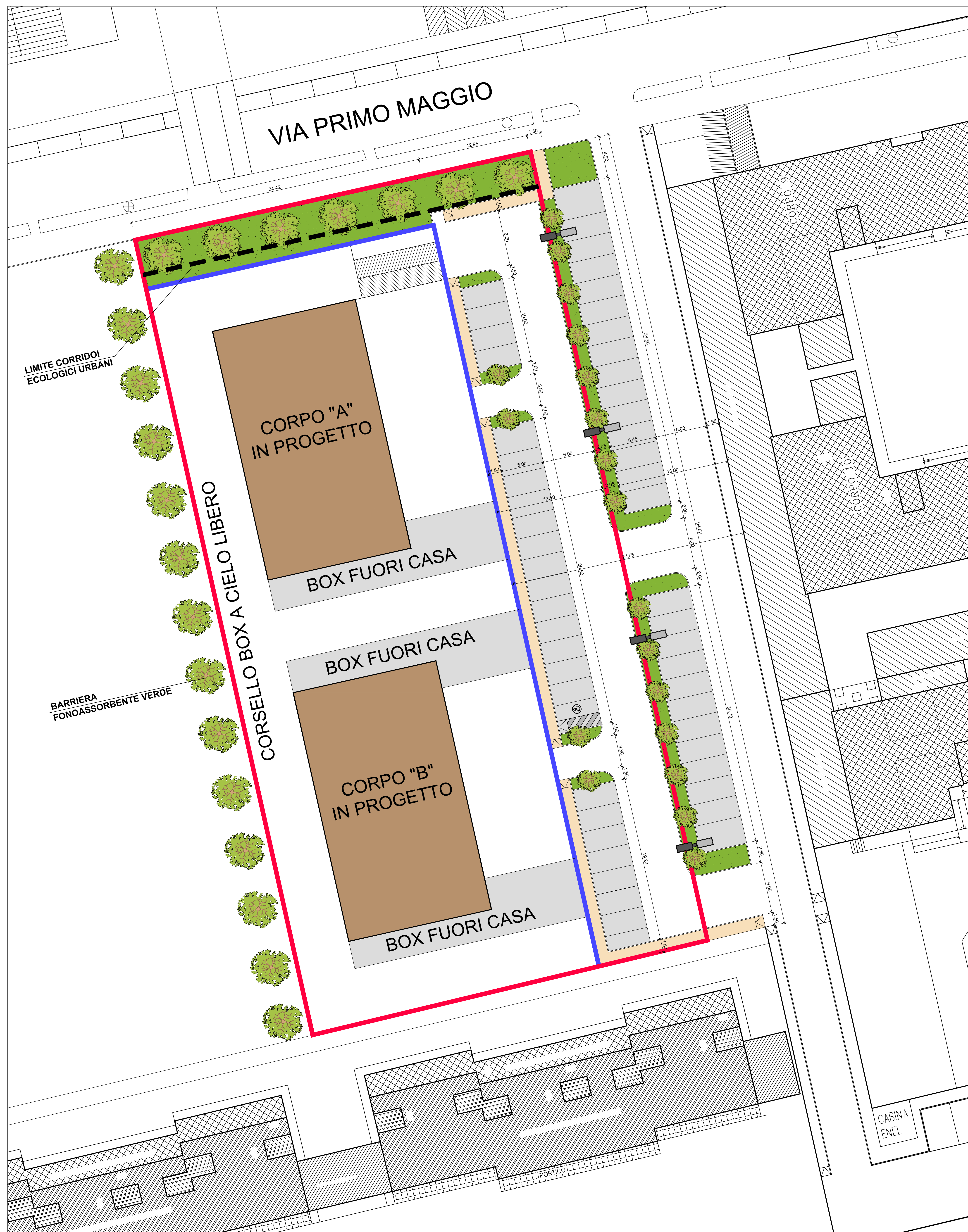
PLANIMETRIA GENERALE URBANIZZAZIONI - STATO DI PROGETTO Scala 1:500
